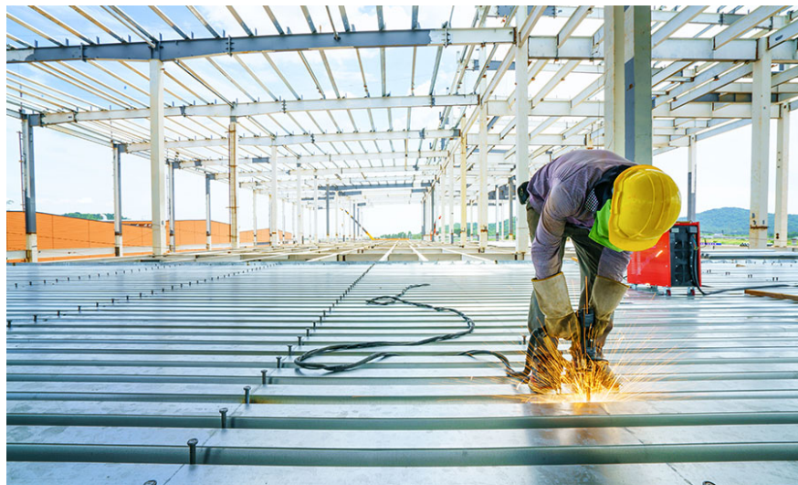
Figura 15: instalación del losacero PSI Concreto
